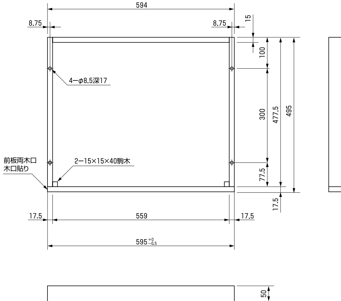
【製品外形図】
