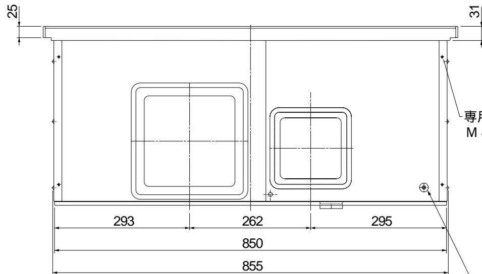
下面図
