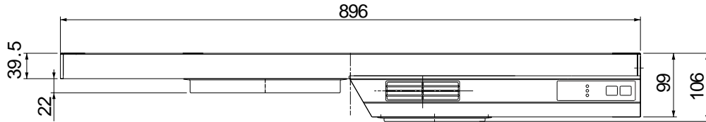
正面図
