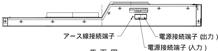
背面図
