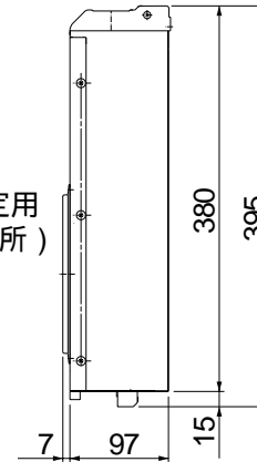
側面図
