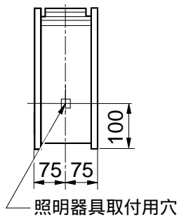
下面図
