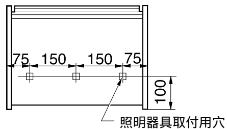
下面図
