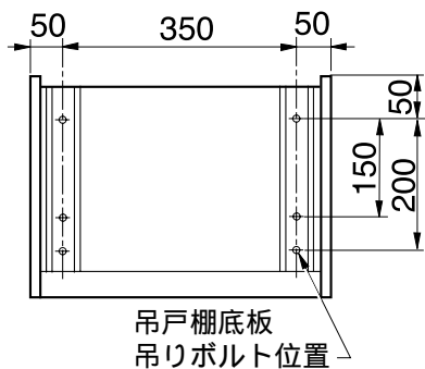
上面図
