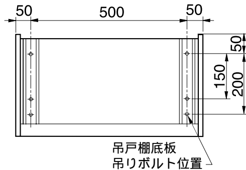
上面図
